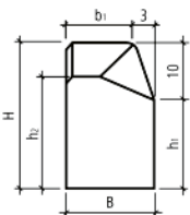
Anschlussrandstein links / rechts b1 = 12 cm h1 = 15 cm
