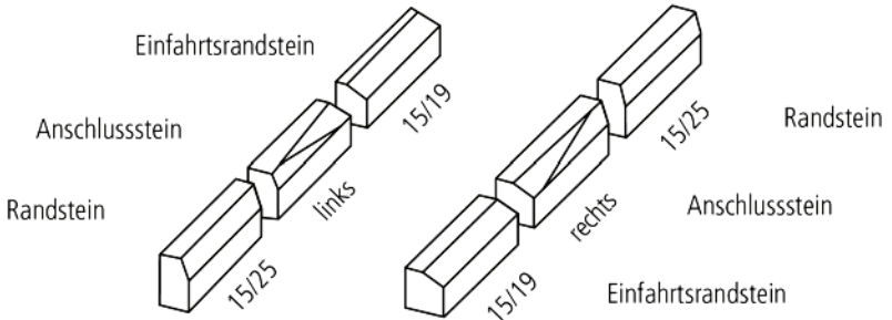
Einfahrtsrandstein b1 = 5 cm h1 = 4 cm
