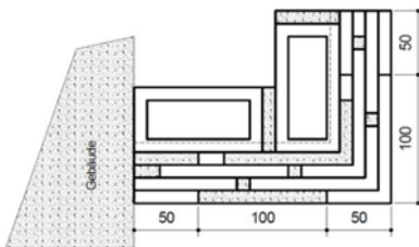
Beispiel 2 (Grundriss)
