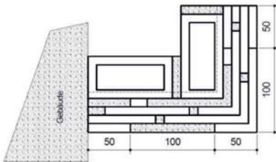
Beispiel 2 (Grundriss)
