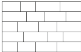
Schichtmauerwerk H 16 cm
